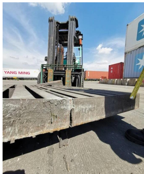
ภาพ : สภาพการวิบัติของคอนกรีต และเหล็กปากฝาท่อ
