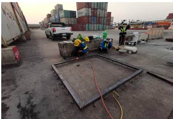
ภาพ : บรรยากาศหน้างาน ภายในลานขนถ่ายสินค้า
