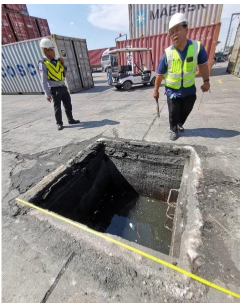
ภาพ : สภาพการวิบัติของคอนกรีต และเหล็กปากฝาท่อ
